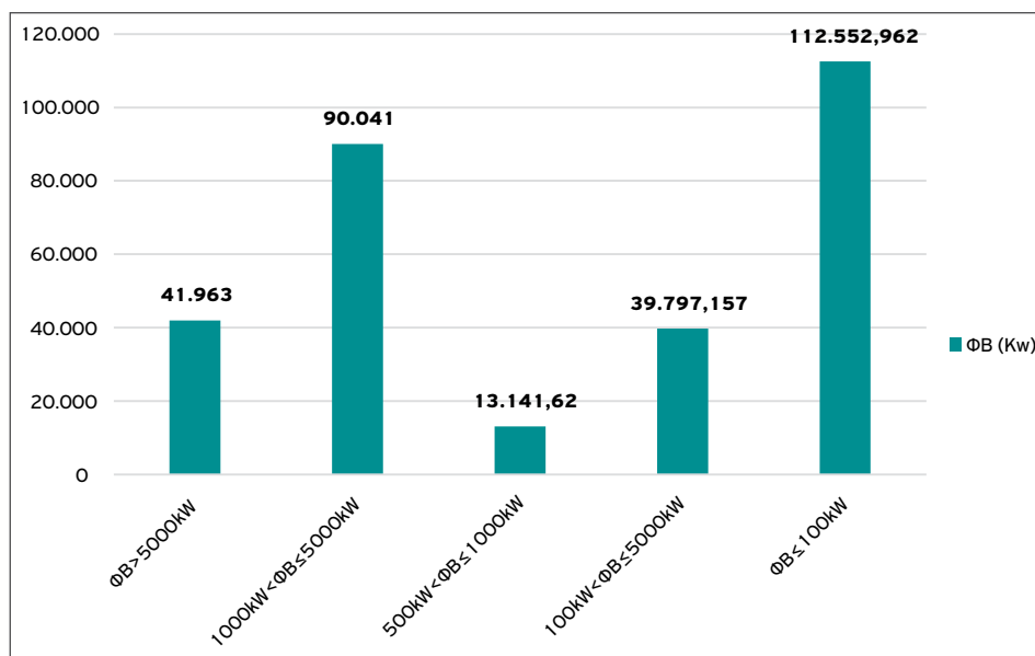
Διάγραμμα 18: Εγκατεστημένη ισχύς (kW) μονάδων ΑΠΕ και ΣΗΘΥΑ φωτοβολταϊκών στην Πελοπόννησο στο διασυνδεδεμένο σύστημα (Νοέμβριος 2017)
