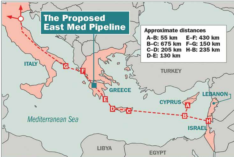
Εικόνα 1: Κατασκευή του διασυνδετήριου αγωγού Eastern Mediterranean Pipeline (East Med) και η διέλευσή του από την Πελοπόννησο
