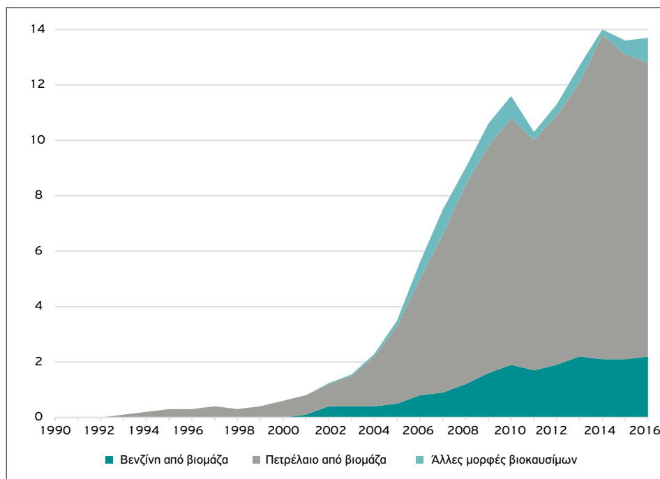
Διάγραμμα 49: Πρωτογενής παραγωγή από ρευστά βιοκαύσιμα (ΕΕ-28, 1990-2016, εκατ. ΤΙΠ)
