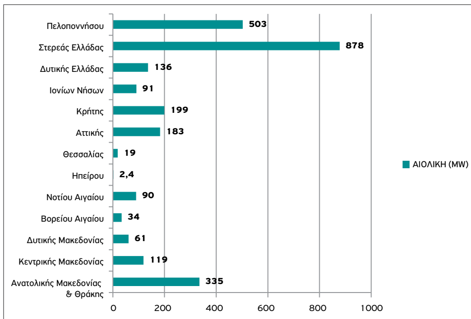
Διάγραμμα 20: Κατανομή αιολικών πάρκων (MW) ανά περιφέρεια
